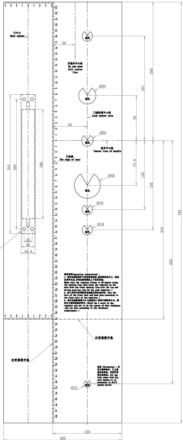
具体尺寸
